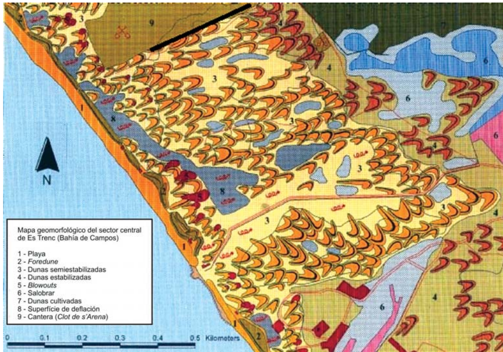
Figura 4. Sector comprendido entre el Clot de s'Arena y es Trenc (parte inferior de la figura). La sección descrita en la paragrafa 3 (ver anexo 2.1) se representa por medio de una línea continua en la parte superior de la figura.
